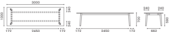
W3000×D1000×H700
