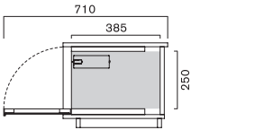
断面図 A-A
