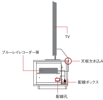
断面図(側面)
