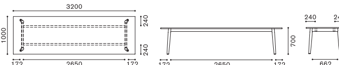
W3200×D1000×H700
