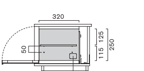
断面図 B-B
