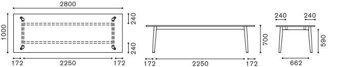
W2800×D1000×H700
