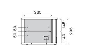
断面図 C-C
