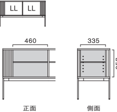
LLタイプ (W460)
