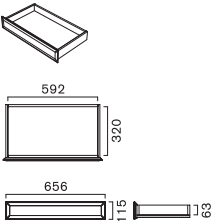
Lタイプ (W656)
